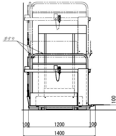
B詳細図
