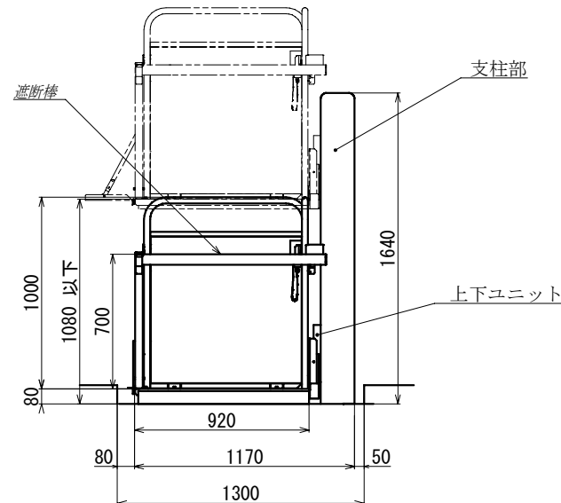
A詳細図
